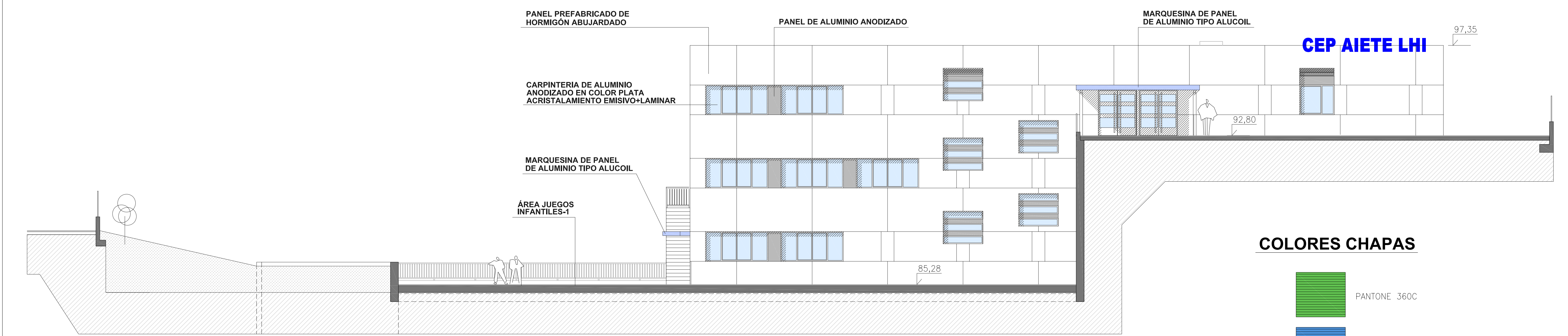
ALZADO NORTE
