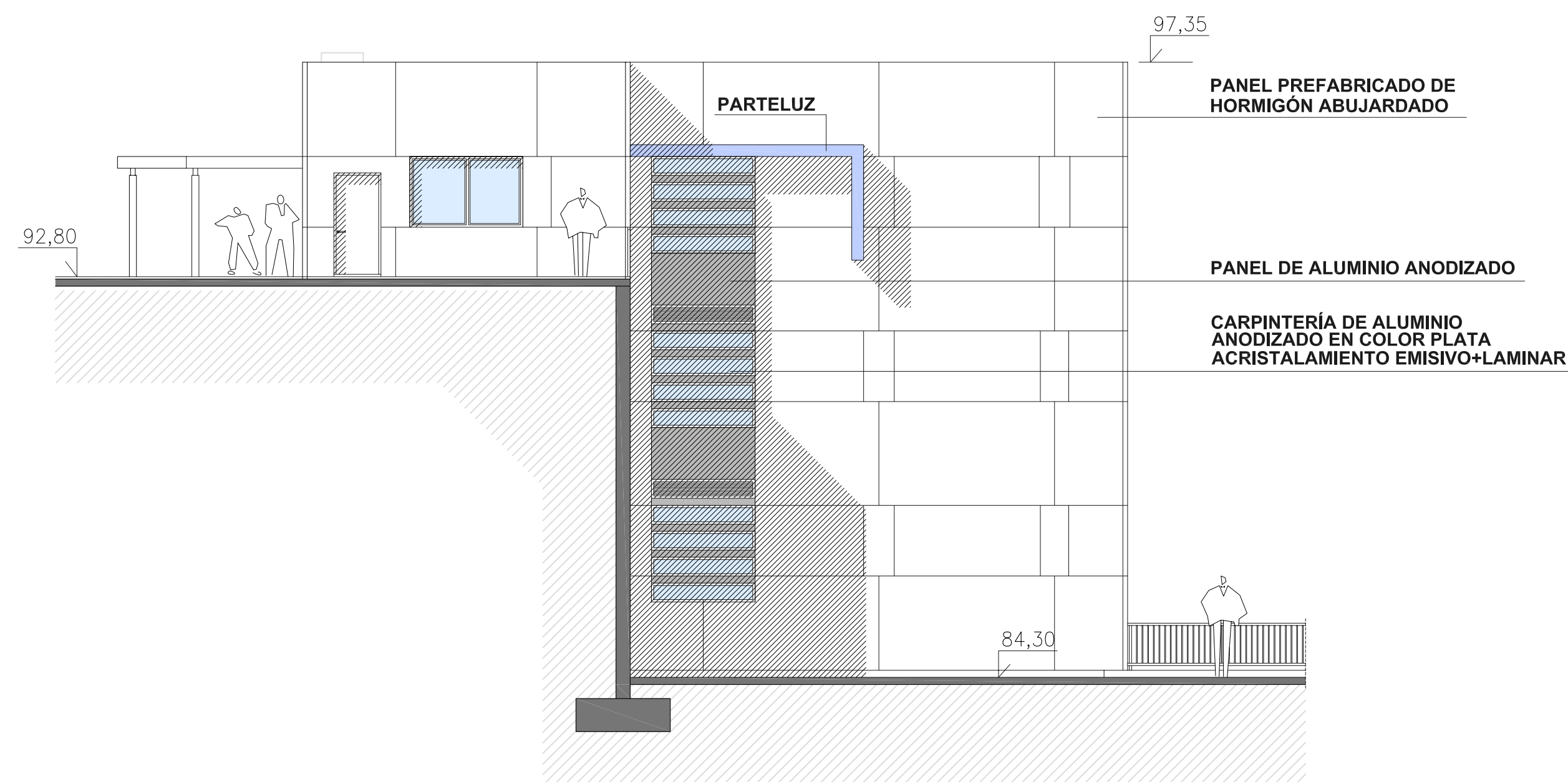
ALZADO OESTE
