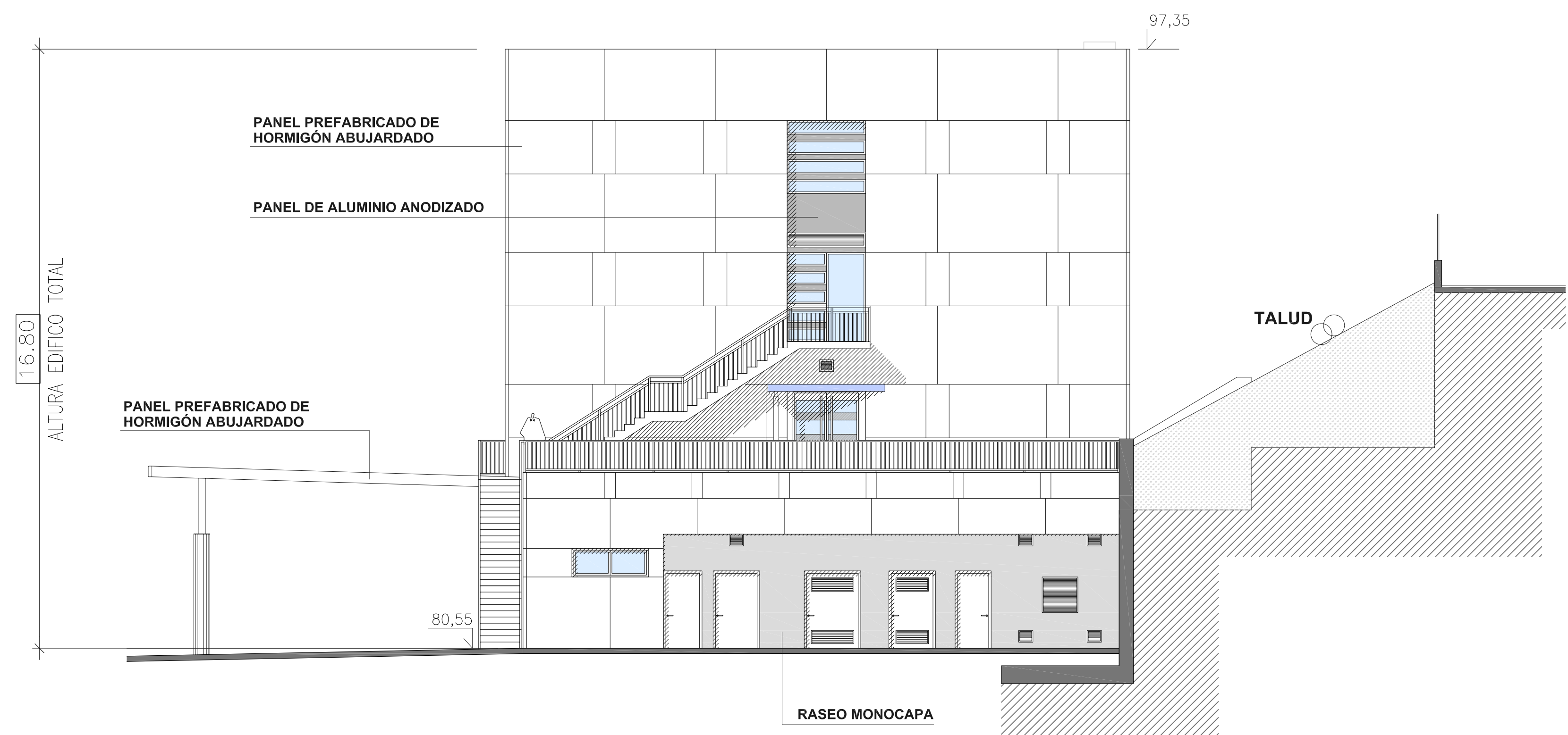
ALZADO ESTE
